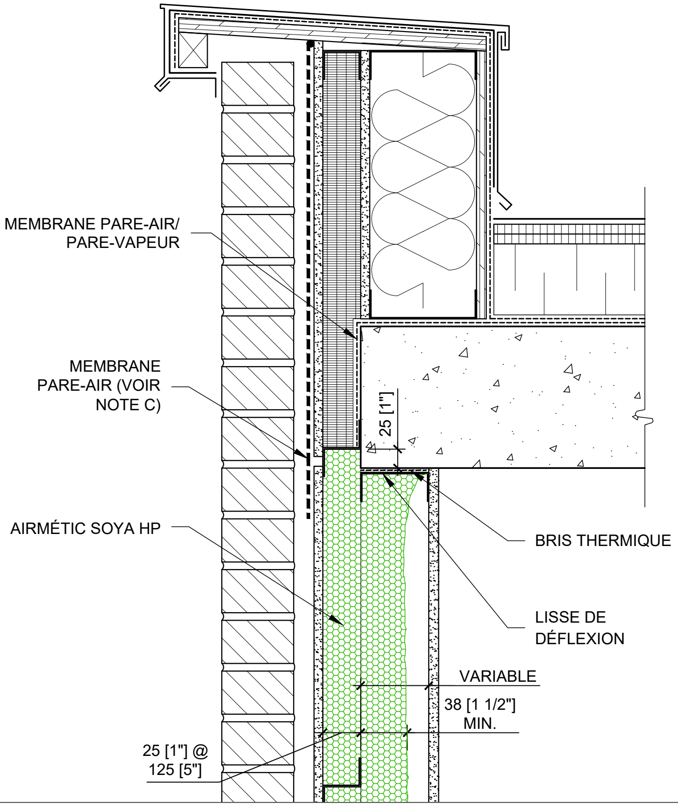
PARAPET / AIRMÉTIC SOYA HP INTÉRIEUR POUTRE REVÊTEMENT DE BRIQUE
