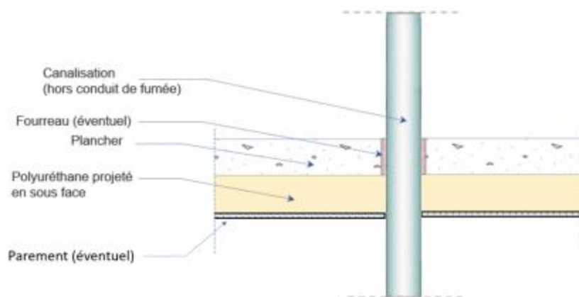
Figure 4 : Traitement d'une canalisation verticale
