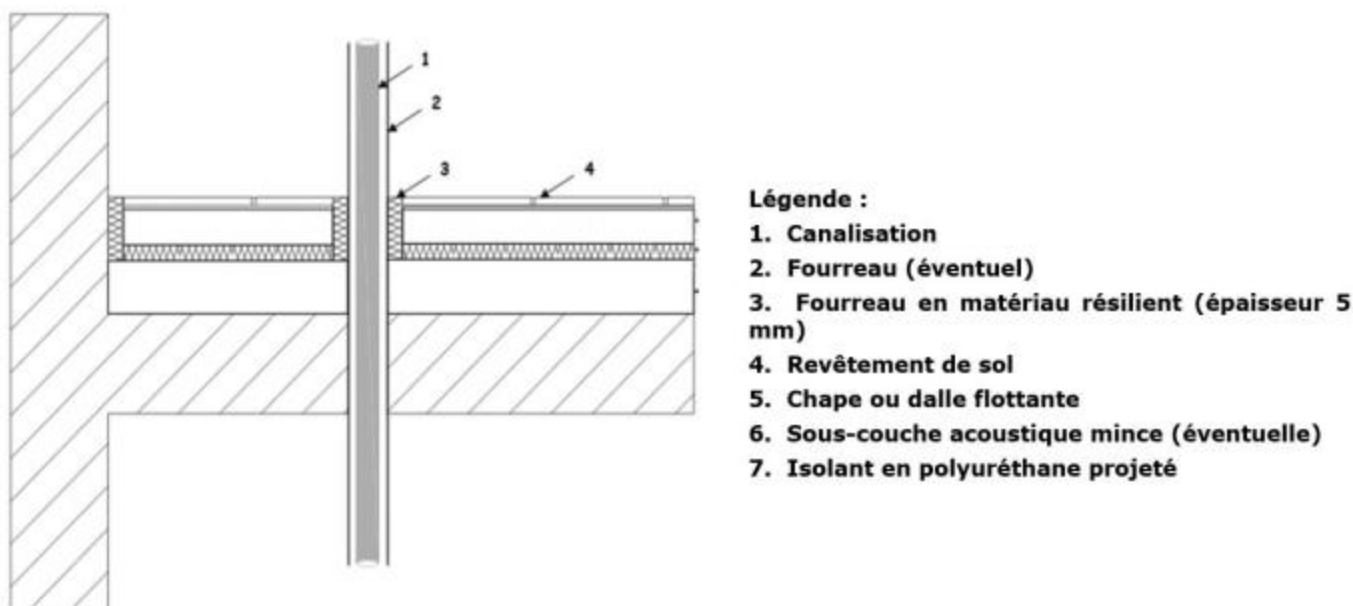
Figure 5 : Traitement d'une canalisation verticale traversant le support
