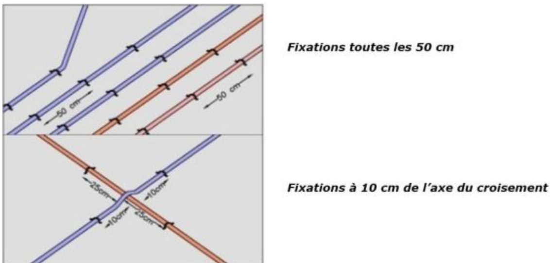
Figure 4 : Traitement des canalisations
