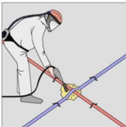
Figure 6 : Projection sur les croisements de gaines
